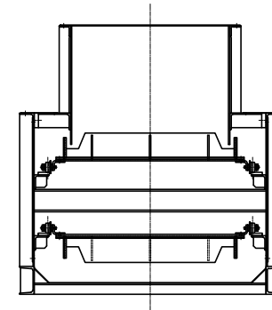
中間断面図 S=1/15
