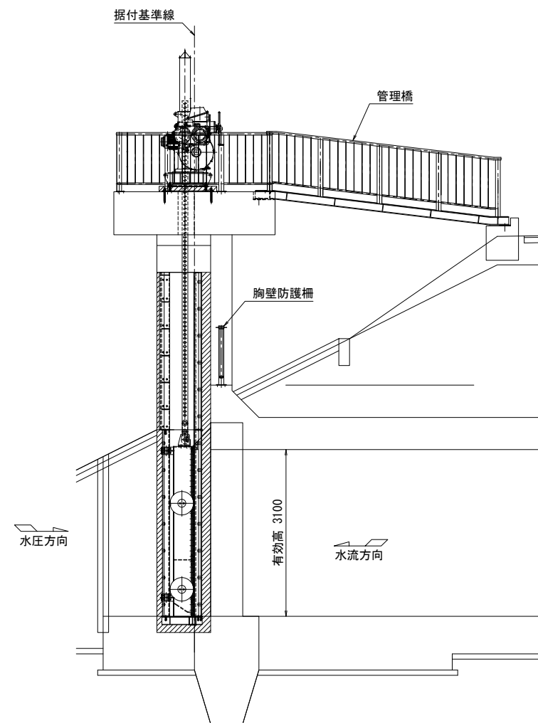
側面図 S=1:50
